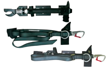
耐衝撃性40G 万能! 頑丈! 怪力! TG3033 ¥220,000 (税込¥242,000) 本体 重量4.2kg オノ部2.6kg 鈎爪部1.6kg 長さ565mm (収納時) 840mm (伸長時) 材質特殊合金スエーデン鋼 救助・運搬 兼用ベルト 重量0.85kg 長さ2500mm 材質ポリエステル 破壊荷重 ベルト>30kN D環、フック・バックル>20kN スタンド (ホルダー) 材質アルミニウム3mm 90×453×53mm 0.45kg
